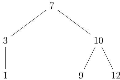
Figura 3.2: Albero binario di ricerca
